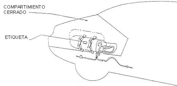
Fig6.- Cilindro instalado en compartimento cerrado
