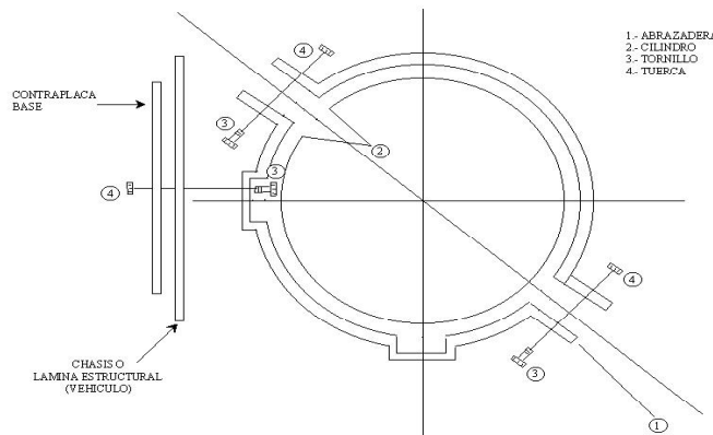
Figuras 4. Abrazadera para recipiente de GNC
