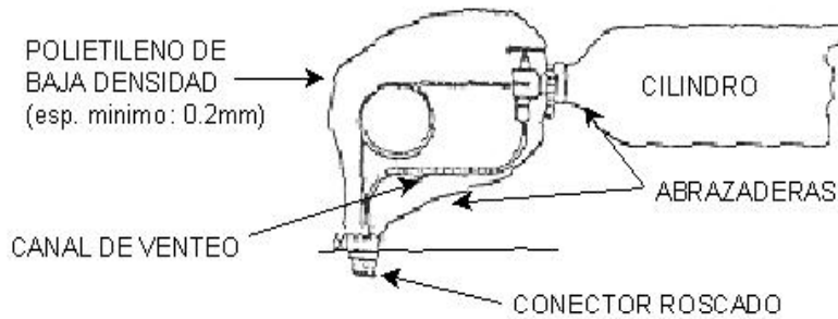
Figura típica 7.- Cubierta a prueba de fugas en compartimiento cerrado
