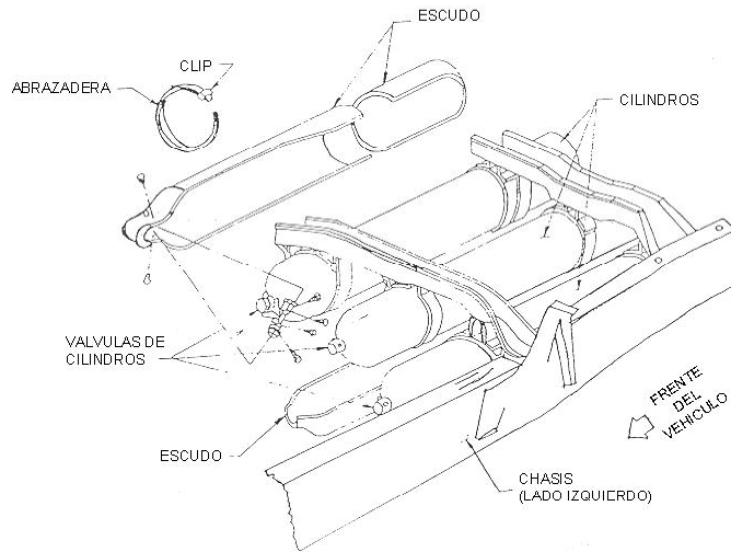
Figura típica 3.- Escudo protector de cilindros
